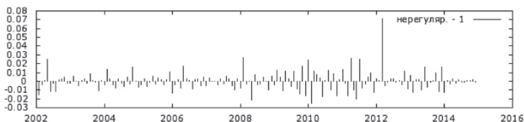
Рис. 4. График случайной составляющей временного ряда уровня безработицы
