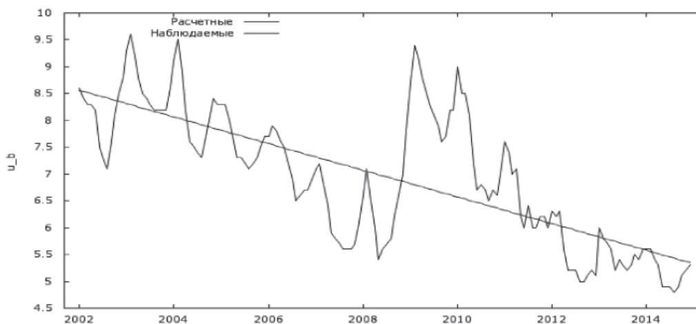
Рис. 1. Фактические данные и график линейного тренда уровня безработицы
