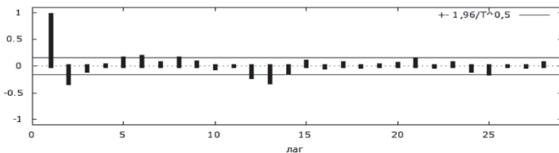
Рис. 5. График зависимости значений частной автокорреляционной (PACF) функции от величины лага
