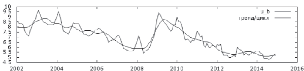
Рис. 3. Графики исходного ряда и тренд-циклической компоненты
