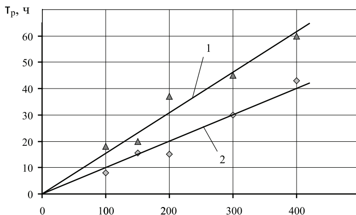
Рис. 3. Зависимость равновесного времени обезвоживания шейхцерицево-сфагнового торфа степенью разложения 22...25% (при учете гравитационного потока влаги и испарения) от начальной толщины слоя (конвективный теплоподвод – 1, радиационно-конвективный теплоподвод – 2) \tau_{pi} = k_{hi} \cdot h_n , k_{hi} = 0,15 \cdot 10^3 ч/м, k_{h2} = 0,1 \cdot 10^3 ч/м
