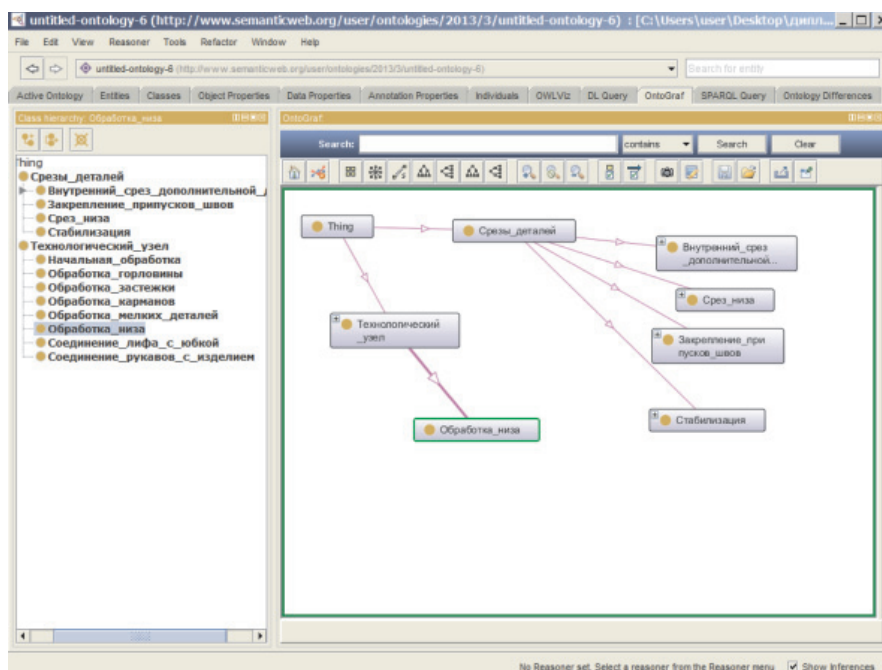
Рис. 4. Диалоговое окно программы Protégé 4.2 beta: экземпляры подкласса «Внутренний срез дополнительной детали» класса «Срезы деталей»
