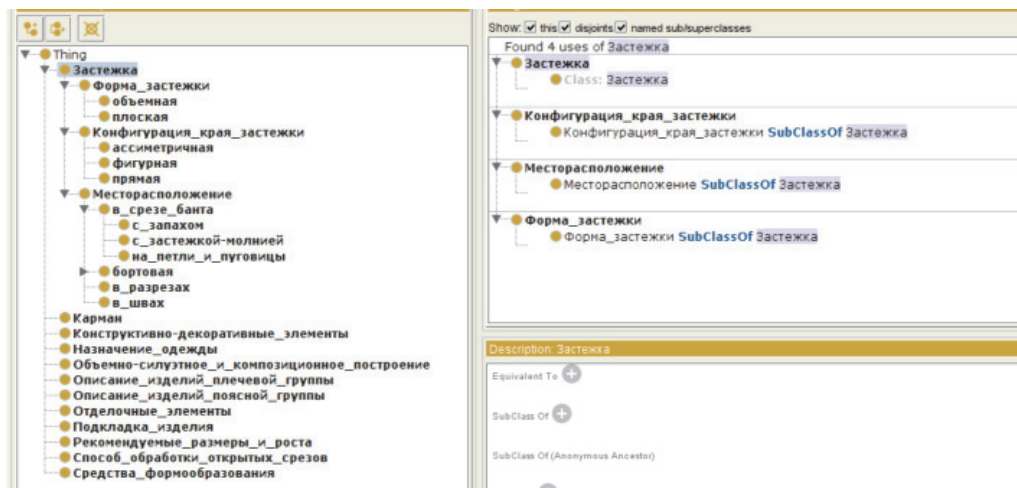
Рис 2. Классификация структуры онтологической модели «Описание проектируемого изделия» (на примере класса «Застежка»)
